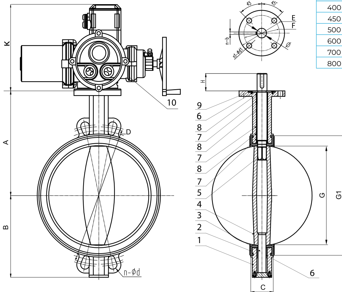
Размеры шпонки
