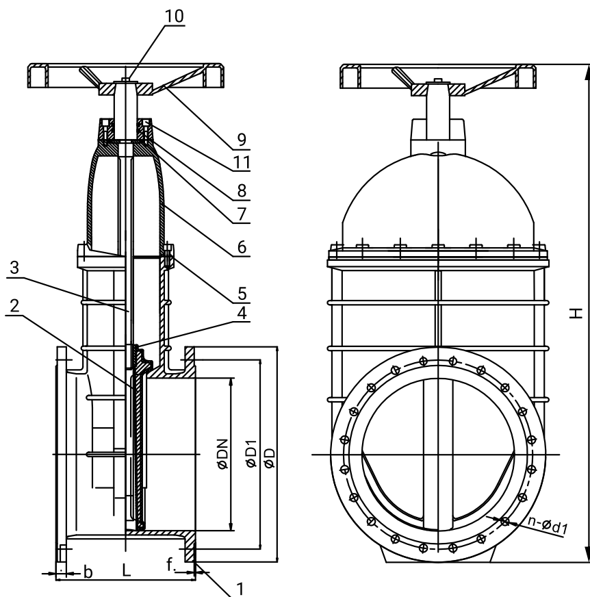
DN350-600
